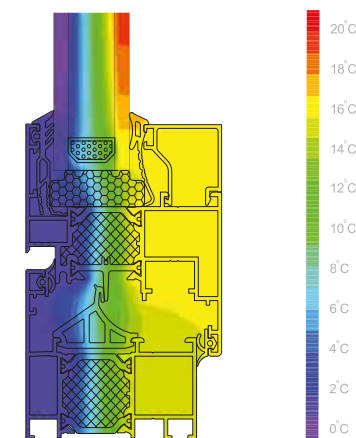
4600i 2 Multilock Διάγραμμα Ισοθερμικής Ροής
