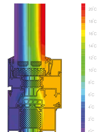
XCLUSIVE 86i 2 Multilock Διάγραμμα Ισοθερμικής Ροής
