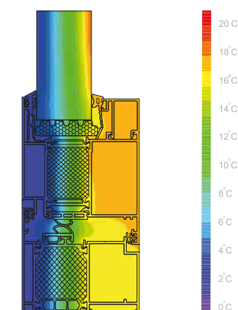
XCLUSIVE 88i² | Κύρια Είσοδος Διάγραμμα Ισοθερμικής Ροής
