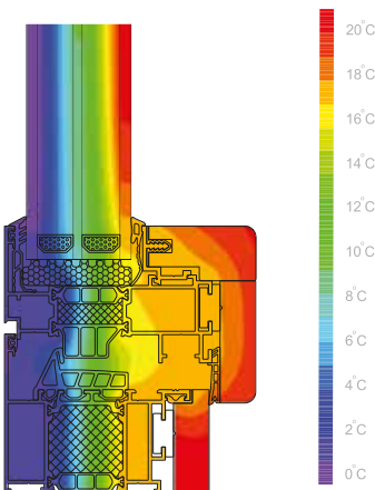
XCLUSIVE 87i² Αλουμίνιο + Ξύλο Διάγραμμα Ισοθερμικής Ροής
