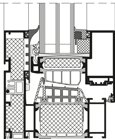
Passivhauszertifizierte Wärmedämmung, Maßstab 1:2,5 Passive house-certified thermal insulation, scale 1:2.5
